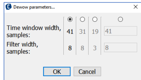
Figure 33 Dewow parameters
